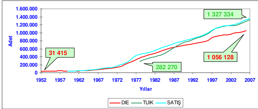
Şekil 4. Türkiye Traktör Parkı Tarihsel Gelişimi
